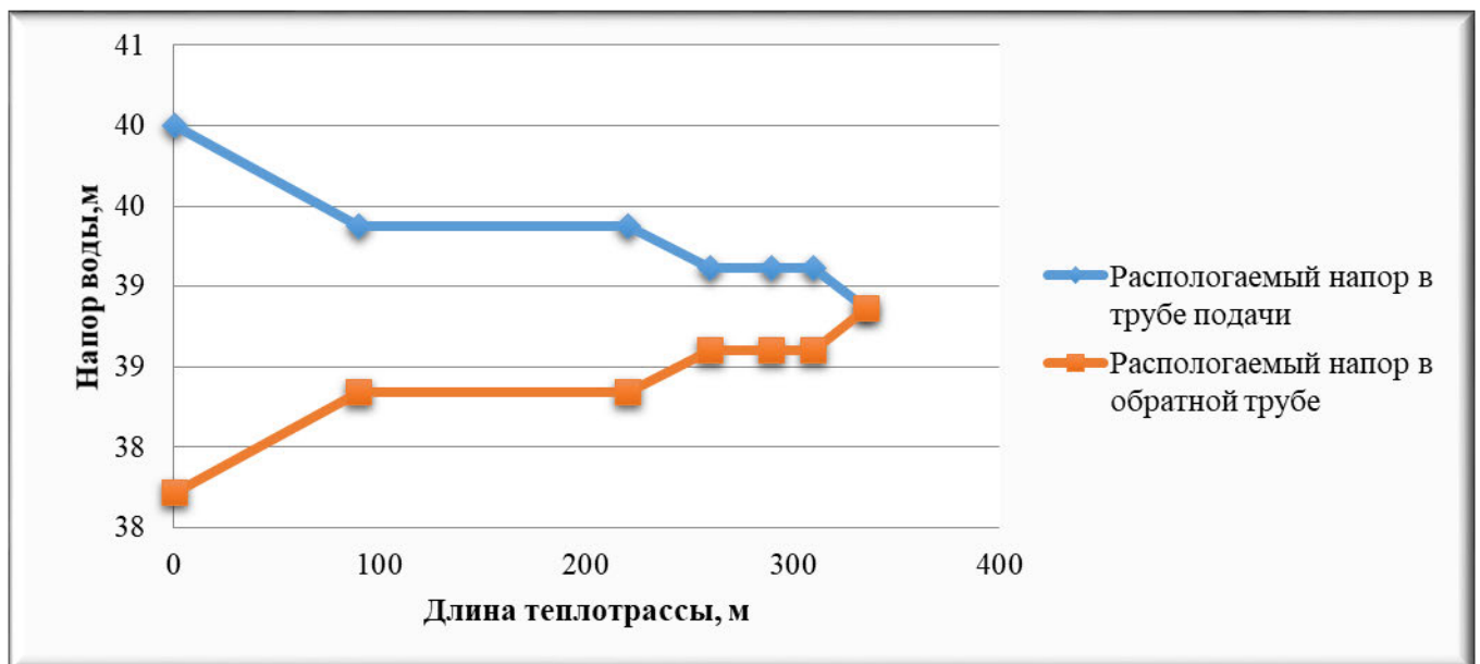
Рисунок 2.5 – Пьезометрический график тепловой сети сельской котельной с. Архангельское по магистральному выводу
