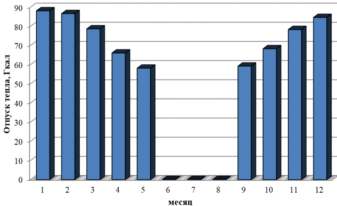
Рисунок 1.2 – Оптимальный температурный график отпуски тепловой энергии для сельской котельной Архангельского сельского поселения
