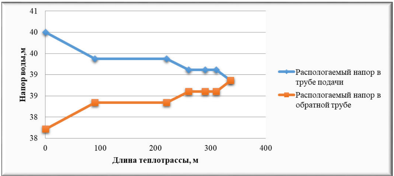
Рисунок 2.4 – Пьезометрический график тепловой сети сельской котельной с. Архангельское по магистральному выводу
